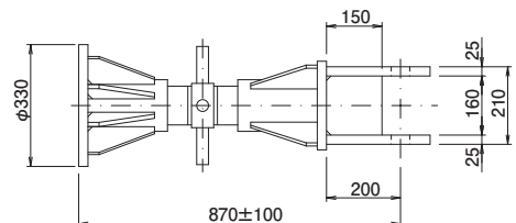
ターンバックル端部詳細図
