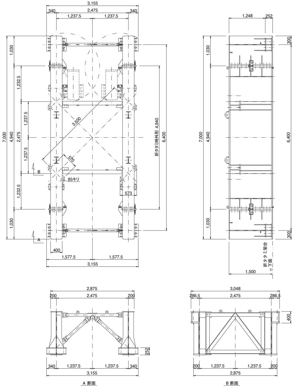
■主要寸法図 (単位：mm)
