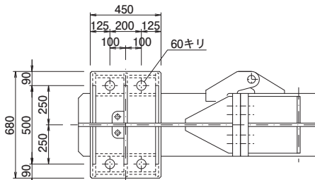
折タタミ架台端部 詳細図
