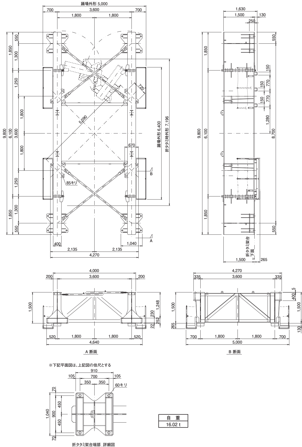
■主要寸法図 (単位：mm)
