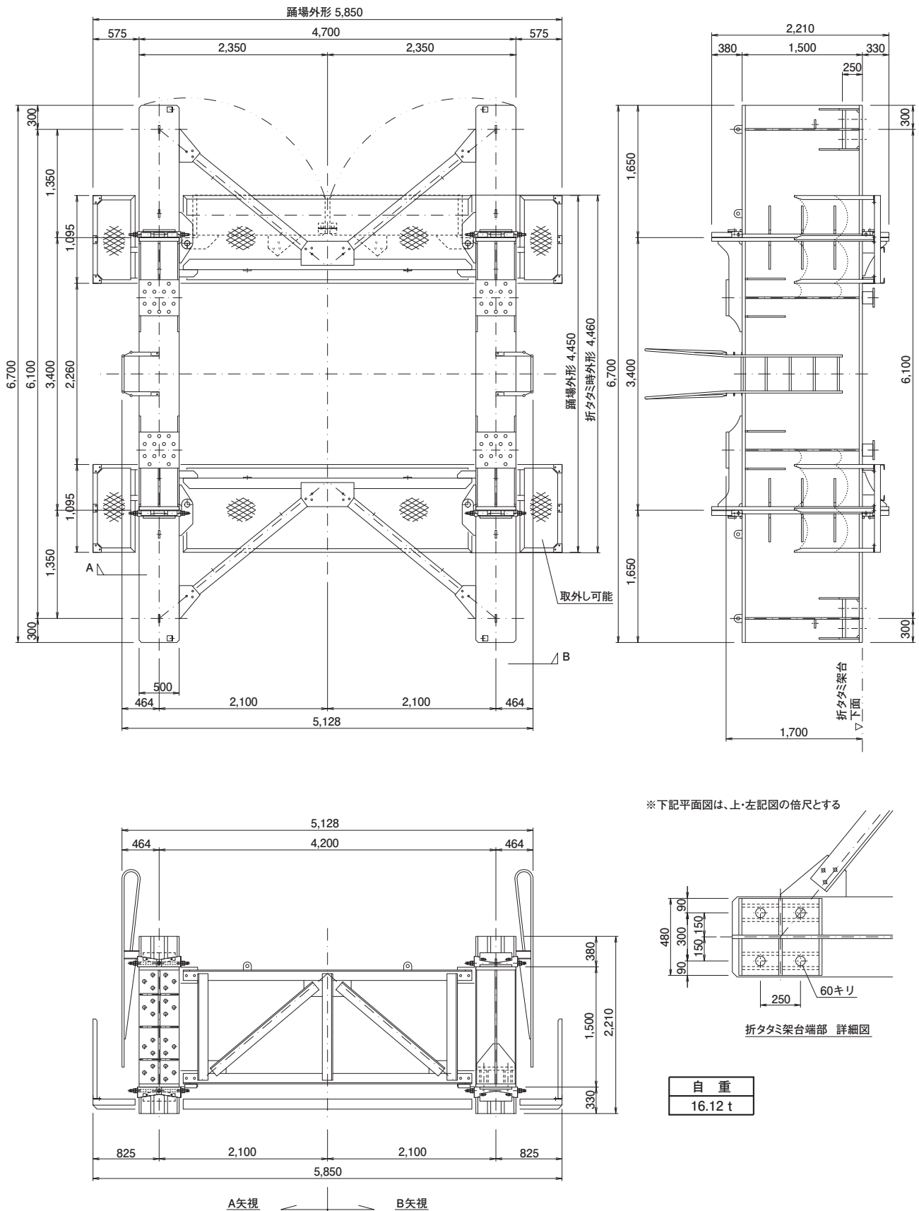
■主要寸法図 (単位：mm)
