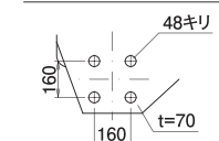
下部盛替梁接合部詳細図
