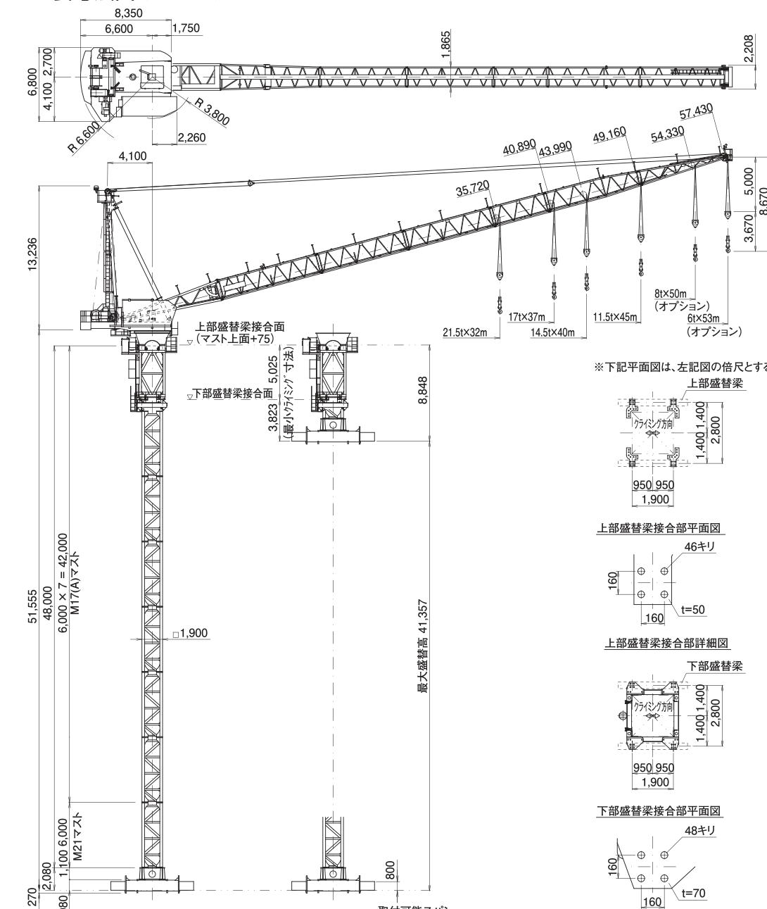
下部盛替梁接合部詳細図
