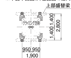
上部盛替梁接合部平面図
