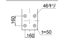
上部盛替梁接合部詳細図
