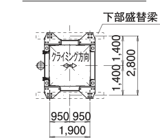
下部盛替梁接合部平面図
