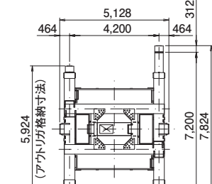
伸縮台座平面図 アウトリガアタッチメント付き (スパン: 7,200 - 6,800)
