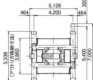
伸縮台座平面図 アウトリガアタッチメント無し (スパン: 6,400 - 6,000)
