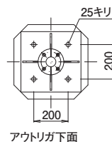
アウトリガ下部 詳細図
