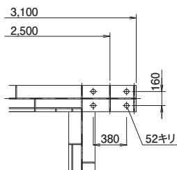
旋回座軸受台端部 下面 詳細図
