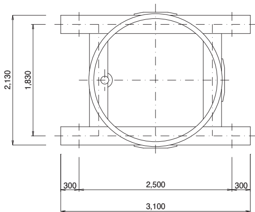
旋回座軸受台 上面 平面図
