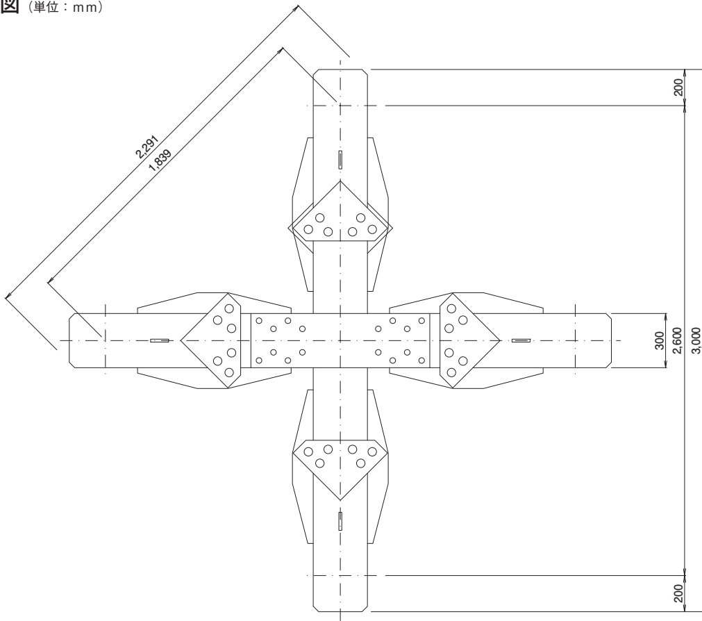
■主要寸法図 (単位：mm)
